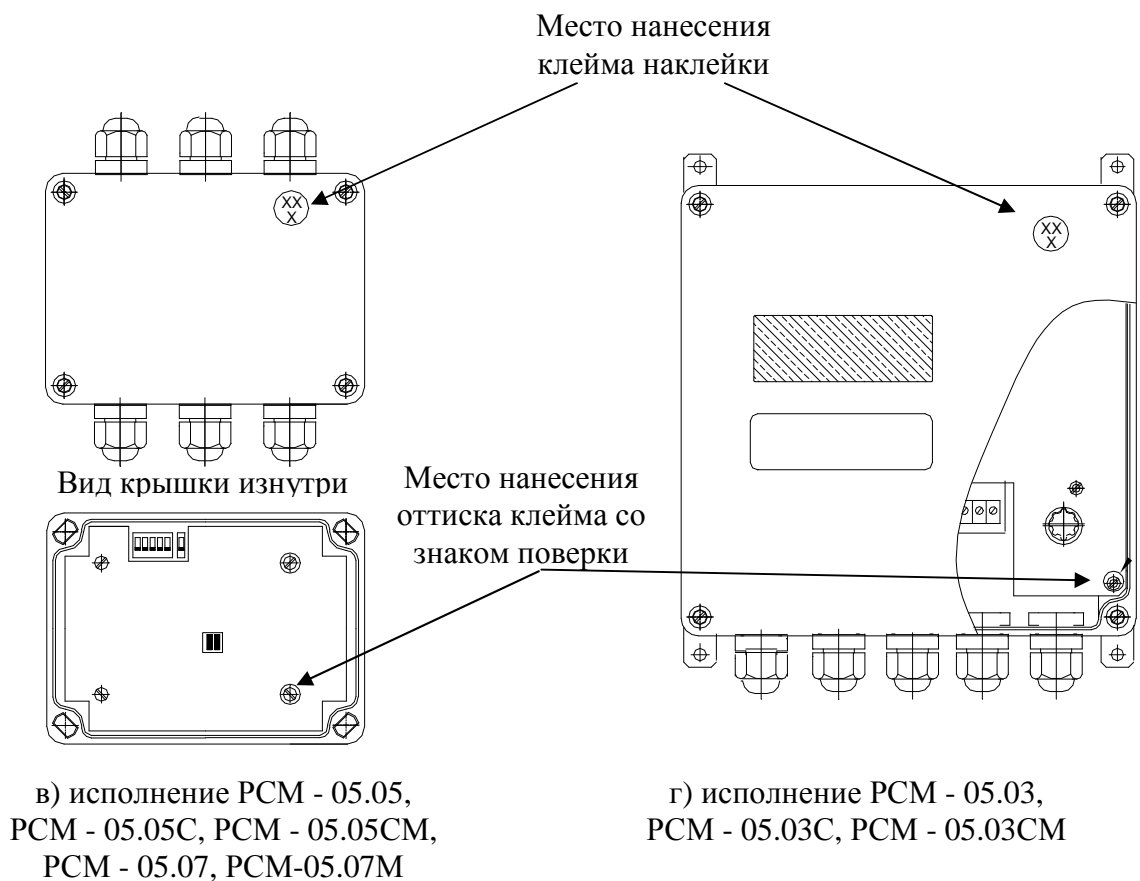
Рисунок 3 – Схема пломбировки расходомеров-счетчиков поверителем
